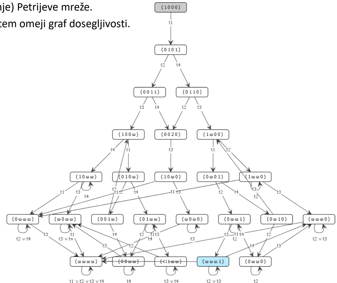
Graf dosegljivosti
